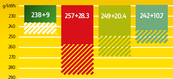
8400R SPOTŘEBA - DIESEL & ADBLUE (DLG POWERMIX)
